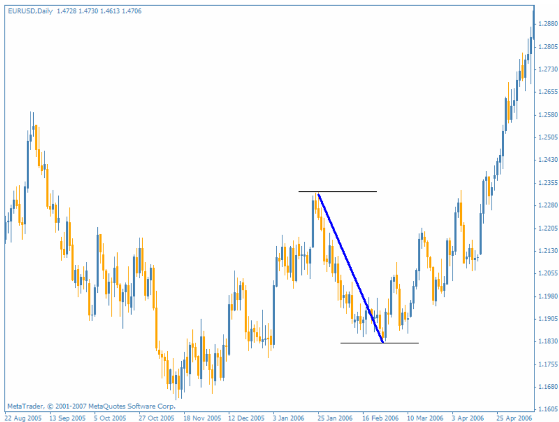
Рис.1. Первое колебание.
