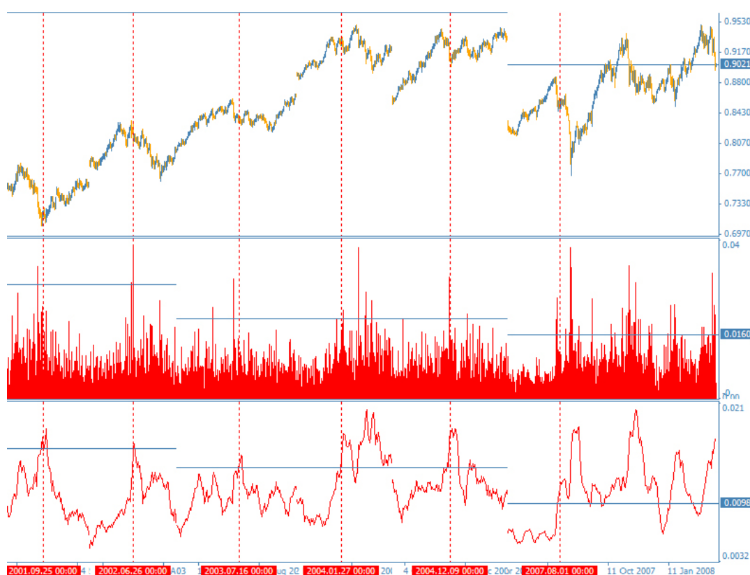
Рис. 1. Волатильность AUDUSD.
