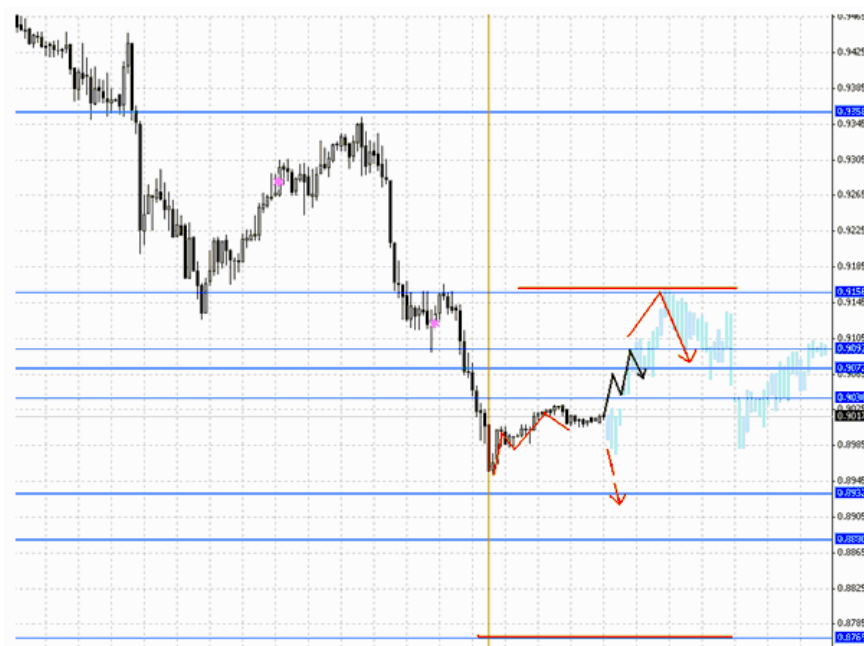
Рис.3. Масштаб Н1.
