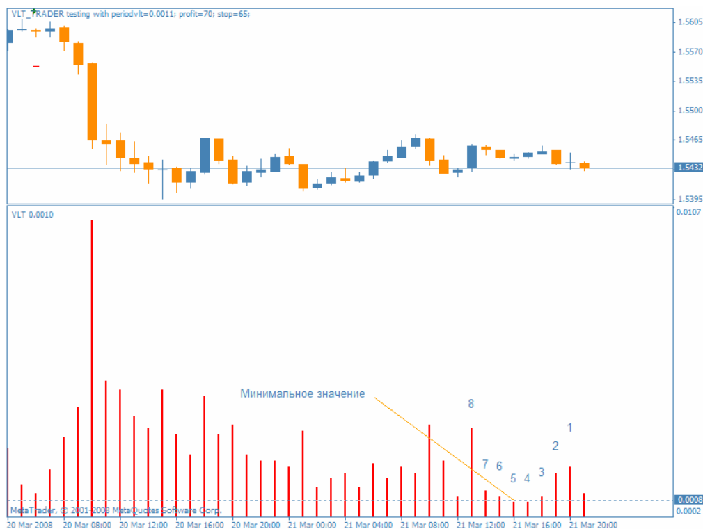
Рис.1. Поиск сигнала.
