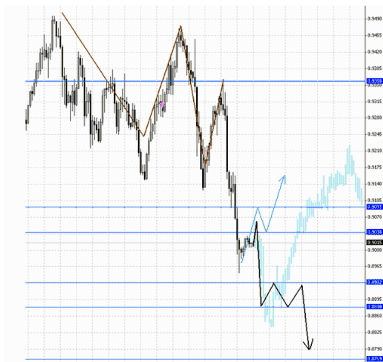
Рис.2. Масштаб H4.
