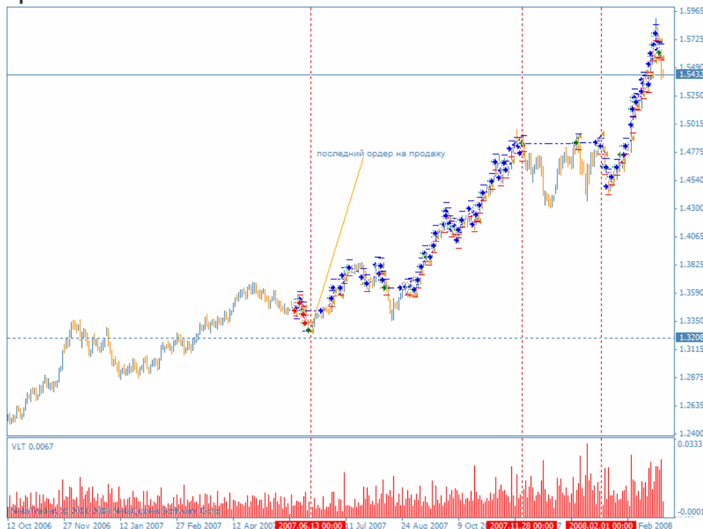
Рис.2. Установка ордеров.
