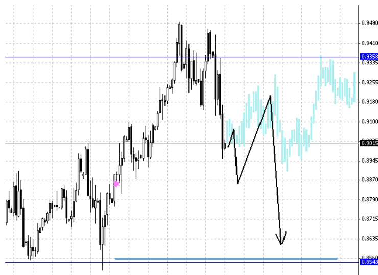
Рис.1. Масштаб D1.
