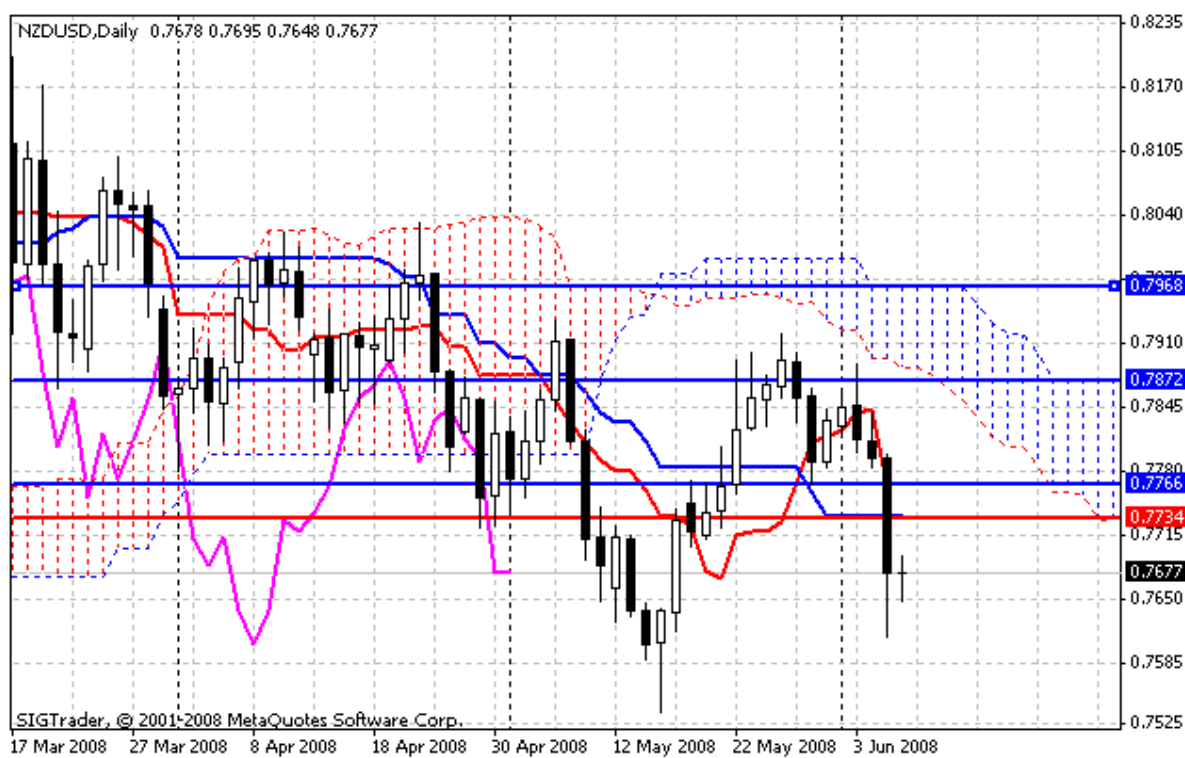
Рис. 2. NZDUSD. Daily.
